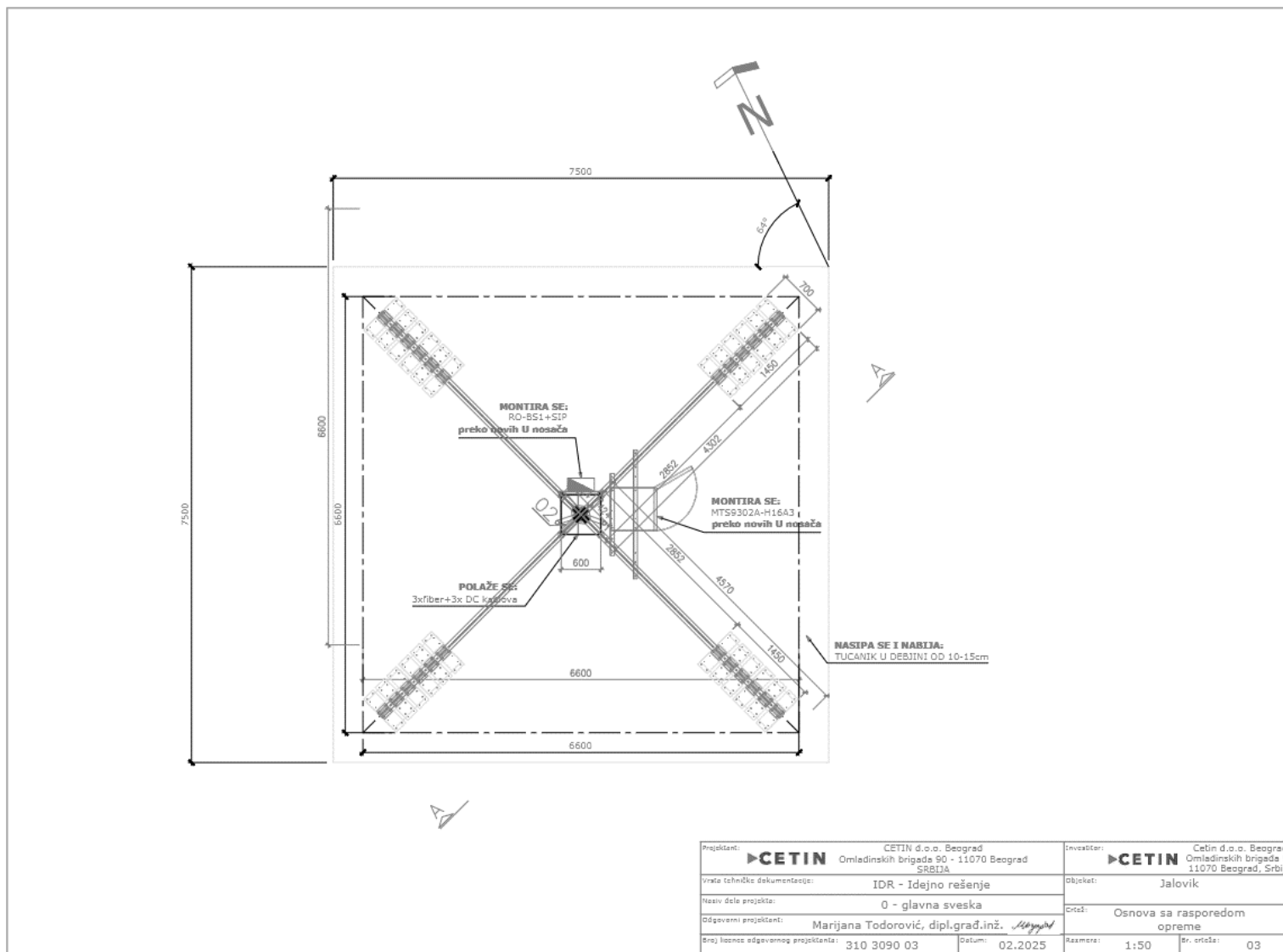
Слика 8.1. Идејно решење – основа стуба са распоредом опреме
