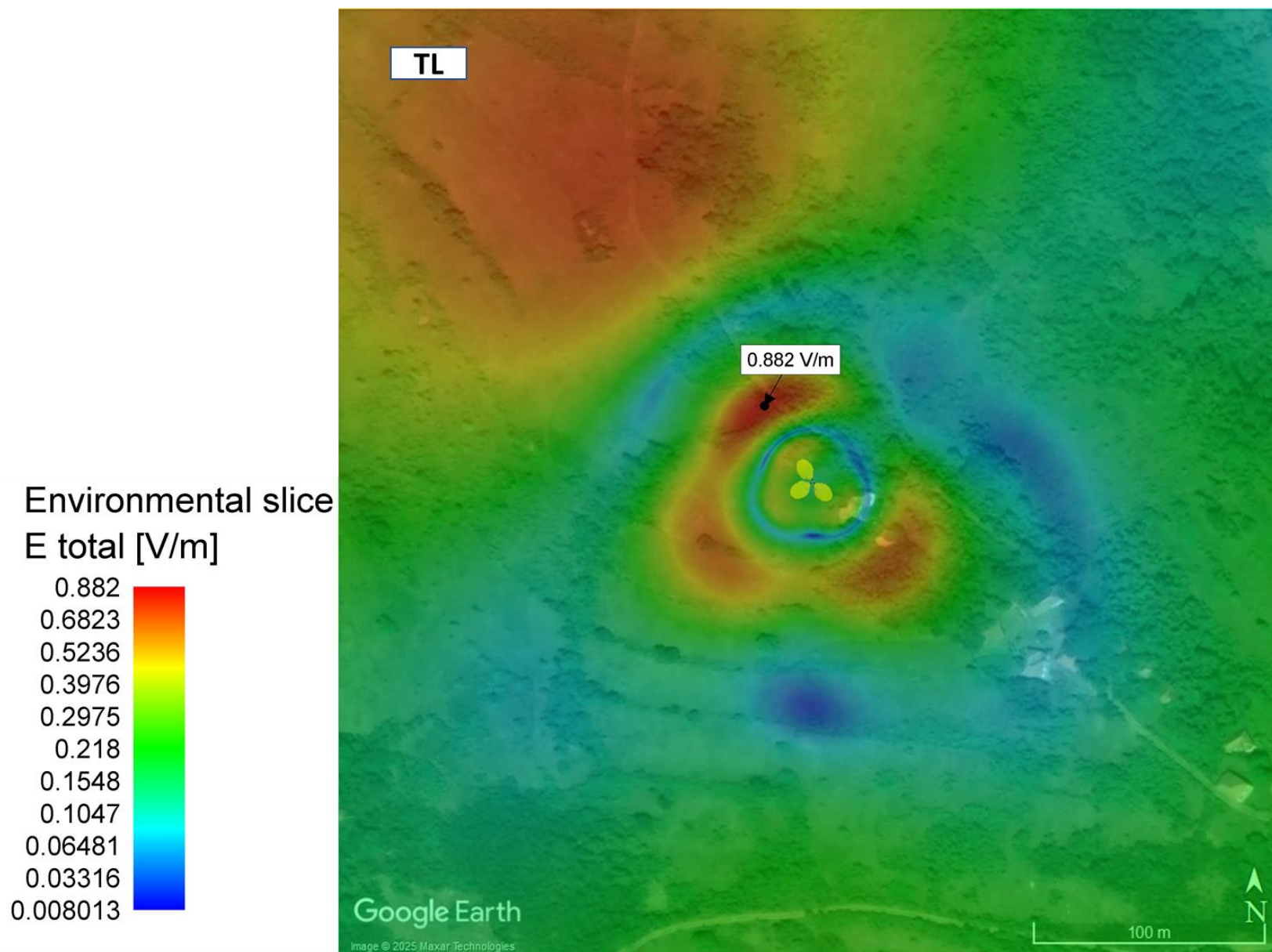
Слика 4.3. Јачина електричног поља на тлу када радио-систем UMTS900 оператора Cetin ради максималним капацитетом
