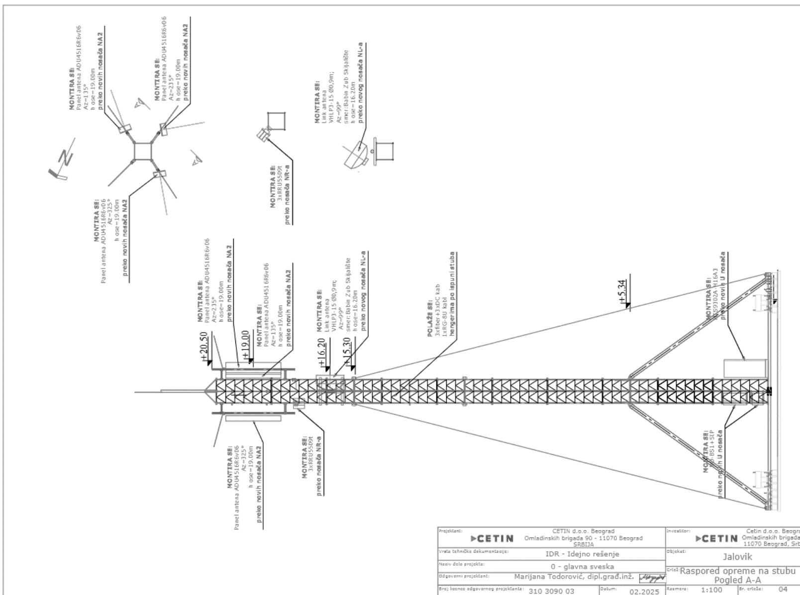
Слика 8.2. Идејно решење – распоред опреме на стубу – поглед А-А
