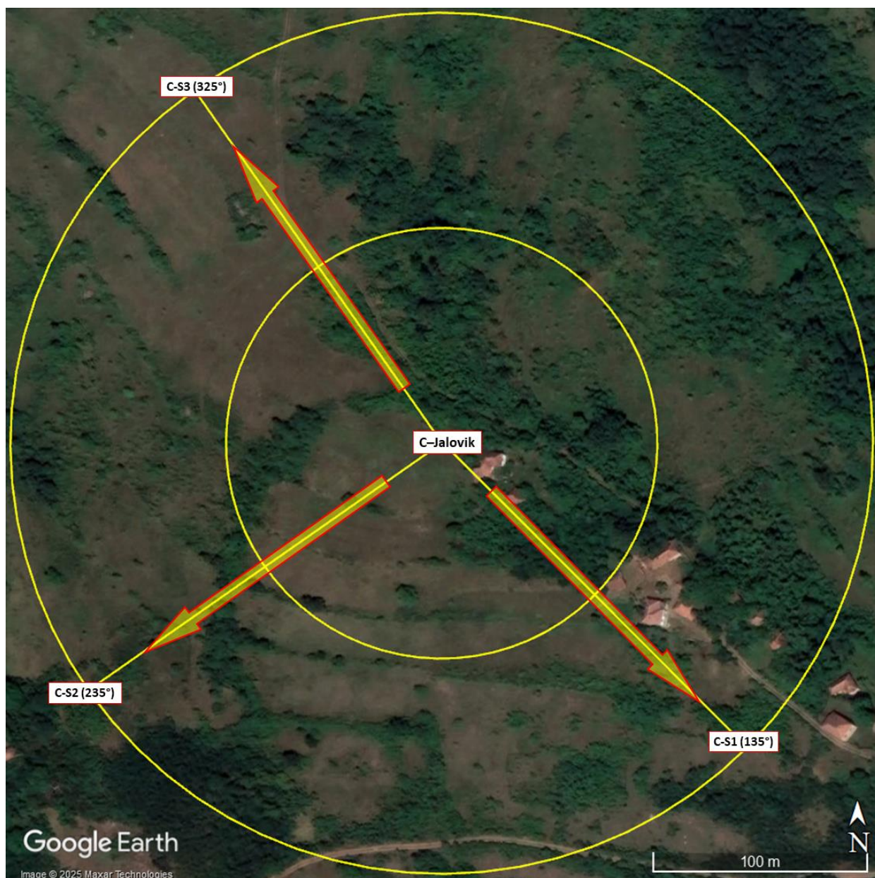
Слика 2.3. Позиција локације са секторима у кругу полупречника 100 и 200 m (са Google Earth)
