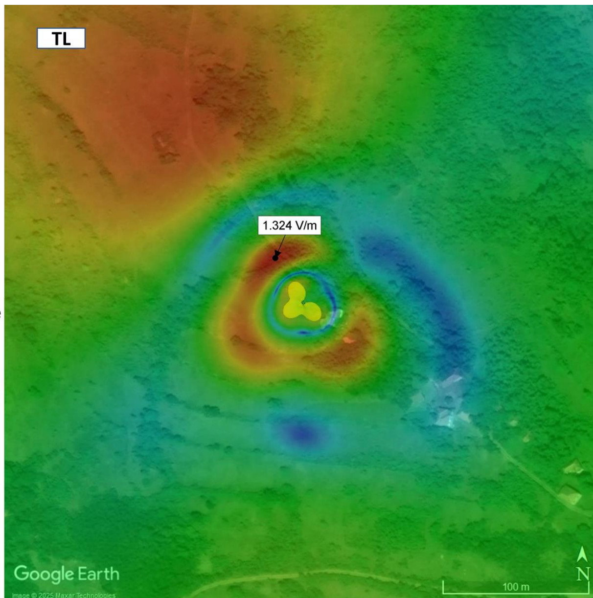
Слика 4.4. Јачина електричног поља на тлу када радио-систем LTE800 оператора Cetin ради максималним капацитетом
